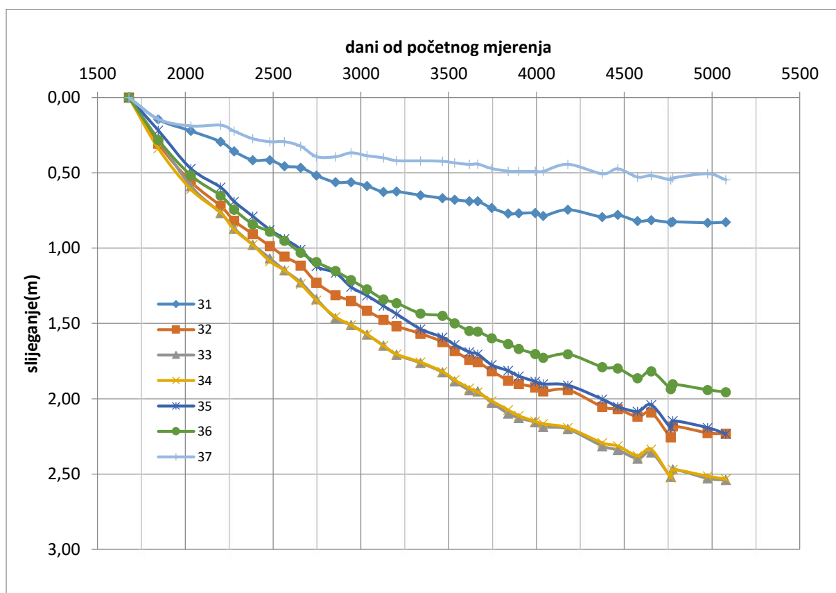
Slika 5. Prikaz konsolidacije repera broj 31, 32, 34, 35, 36, 37 (profil 10). Horizontalna os prikazuje vrijeme u danima a vertikalna os prikazuje slijeganje u metrima. Vrijeme je prikazano u logaritamskom mjerilu. Početni datum mjerenja slijeganja je 30.06.2011
