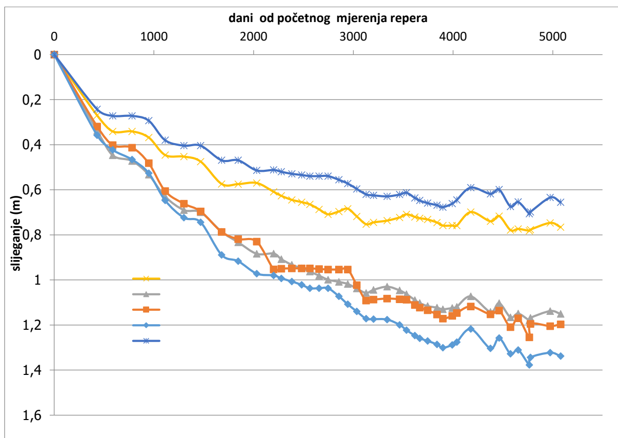
Slika 1. Prikaz konsolidacije repera broj 2, 6, 7, 8, 9 (profil 2). Horizontalna os prikazuje vrijeme u danima a vertikalna os prikazuje sljeganje u metrima. Vrijeme je prikazano u logaritamskom mjerilu. Početni datum mjerenja sljeganja je 24.11.2006.
