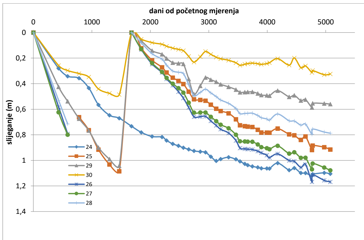
Slika 4. Prikaz konsolidacije repera broj 24, 25, 26, 27, 28, 29, 30. (profil 8). Horizontalna os prikazuje vrijeme u danima a vertikalna os prikazuje slijeganje u metrima. Vrijeme je prikazano u logaritamskom mjerilu. Početni datum mjerenja slijeganja je 24.11.2006. a nakon obnove repera 30.06.2011.
