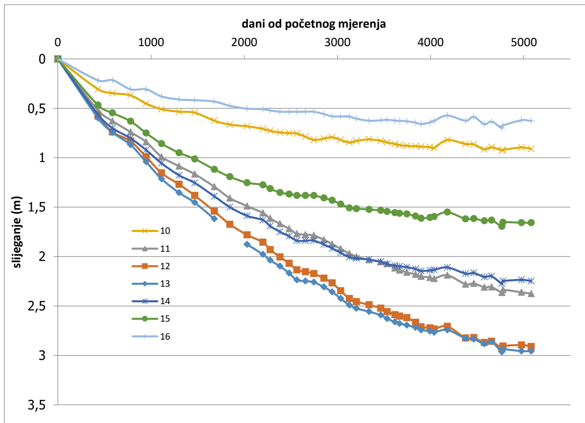
Slika 2. Prikaz konsolidacije repera broj 10, 11, 12, 13, 14, 15, 16 (profil 4). Horizontalna os prikazuje vrijeme u danima a vertikalna os prikazuje slijezanje u metrima. Vrijeme je prikazano u logaritamskom mjerilu. Početni datum mjerenja slijezanja je 24.11.2006.
