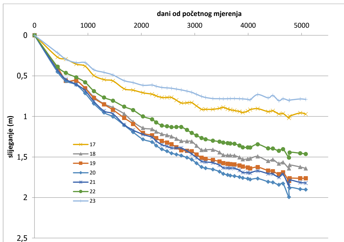
Slika 3. Prikaz konsolidacije repera broj 17, 18, 19, 20, 21, 22, 23 (profil 6). Horizontalna os prikazuje vrijeme u danima a vertikalna os prikazuje slijezanje u metrima. Vrijeme je prikazano u logaritamskom mjerilu. Početni datum mjerenja slijezanja je 24.11.2006.
