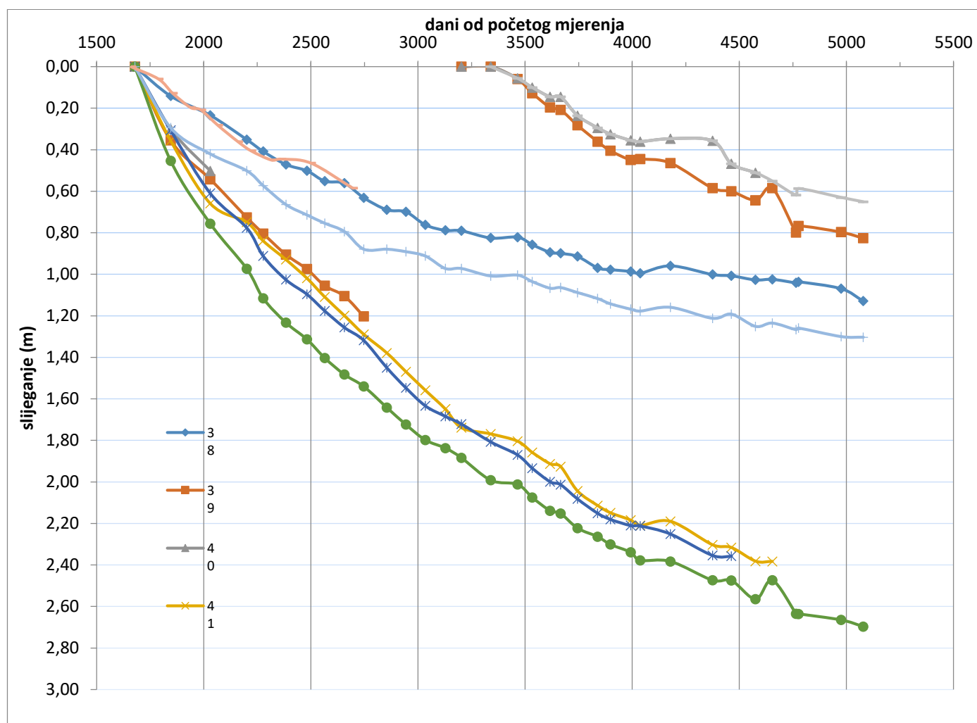
Slika 6. Prikaz konsolidacije repera broj 38, 39, 40, 41, 42, 43, 44 (profil 12). Horizontalna os prikazuje vrijeme u danima a vertikalna os prikazuje slijeganje u metrima. Vrijeme je prikazano u logaritamskom mjerilu. Početni datum mjerenja slijeganja je 30.06.2011.
